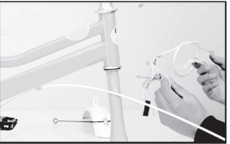
11. ประกอบเบรกหน้าและสายยึดตรรกัว จากนั้นเสียบลอคเข้ากับรูตะเกียบล้อหน้า
