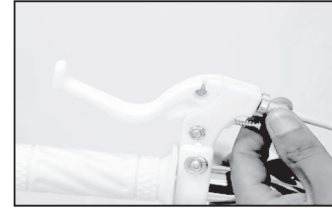
19. ประกอบสายเบรกให้เข้าร่องมือเบรก
