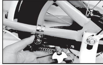
22. หนีบสายเบรกหลังและชันน็อตสายเบรกให้แน่น
